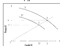
Diagrama para determinar o diâmetro de torneamento.
