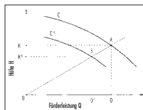
Diagramm zur Bestimmung des Laufraddurchmessers.
