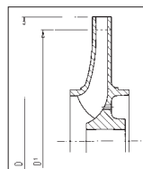
Réduction du diamètre du rouet par tournage.
