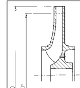
Réduction du diamètre externe du rotor par tournage.
