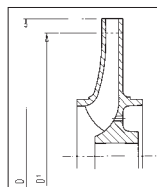
Riducción con tornearo del diámetro exterior del rodete para bomba centrifuga.
